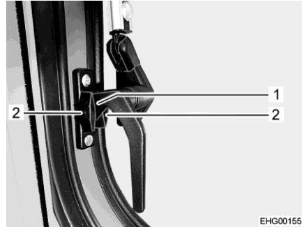
Afb. 52 Vergrendelingshendel, zijkant (stand "continue ventilatie")
