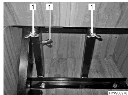
Afb. 30 Tussenstoel met vleugelmoeren vastzetten
