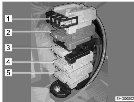
Afb. 127 Zekeringen naast het elektro-blok met voorbereiding voor zonne-energie en satellietinstallatie
