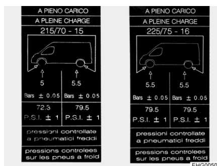
Afb. 188 Aanwijzingssticker voor bandenspanning op B-stijl (voorbeeld)
