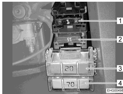
Afb. 121 Zekeringen op de startaccu met laadbooster
