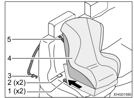
Afb. 16 Bevestiging met Top Tether
