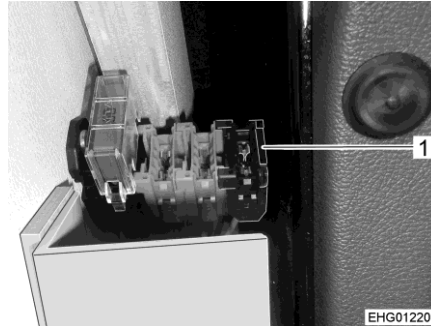
Afb. 132 Zekeringhouder bij voertuig met stuur aan linkerkant (Ford)
