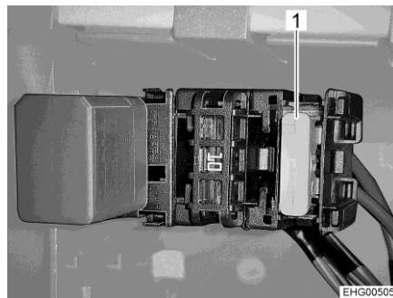
Afb. 128 Zekering op B--stijl, rechterkant van het voertuig (Stellantis)
