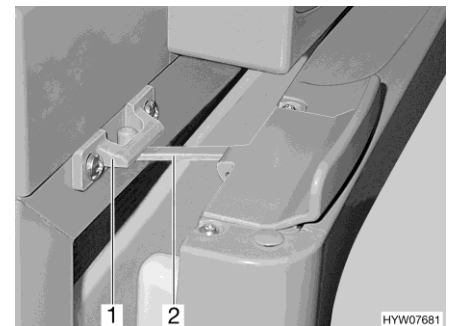
Afb. 151 Koelkastdeur in ventilatiestand (Thetford)
