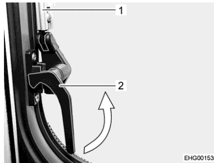
Afb. 48 Vergrendelingshendel, zijkant (stand "gesloten")
