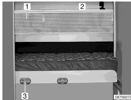
Afb. 90 Veiligheidsnet
