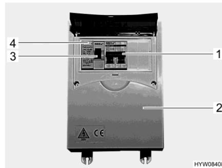
Afb. 116 230-V-zekeringenkast met beveiligingsautomaat en RCD (hoofdschakelaar)
