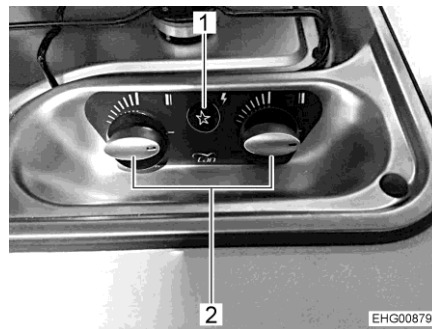
Afb. 143 Bedieningselementen voor gaskooktoestel
