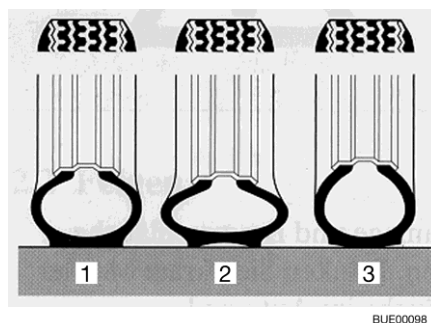
Afb. 187 Draagvlak van de band
