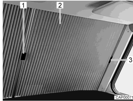
Afb. 7 Vouwverduistering voor voorruit (dicht)
