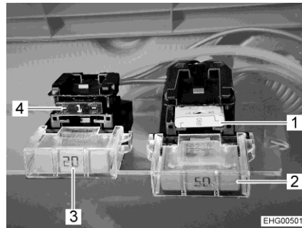
Afb. 123 Zekeringen op de woonruimteaccu met laadbooster (Stellantis)
