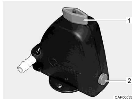
Afb. 153 Veiligheids-/aftapventiel geopend
