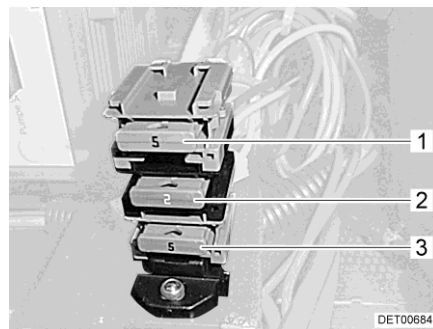
Afb. 125 Zekeringen naast het elektroblok (Stellantis)
