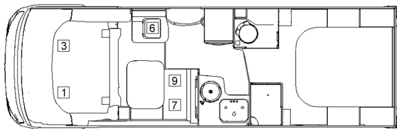
Afb. 17 Zitplaatsen
