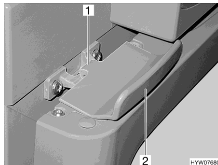
Afb. 150 Vergrendeling van de koelkastdeur, gesloten (Thetford)
