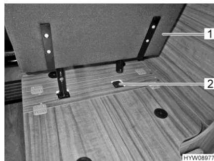
Afb. 29 Tussenstoel in houder steken
