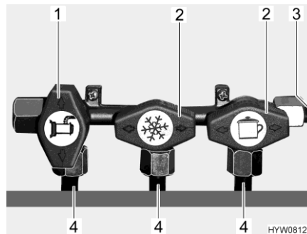
Afb. 111 Stand gasafsluitkranen (voorbeeld)
