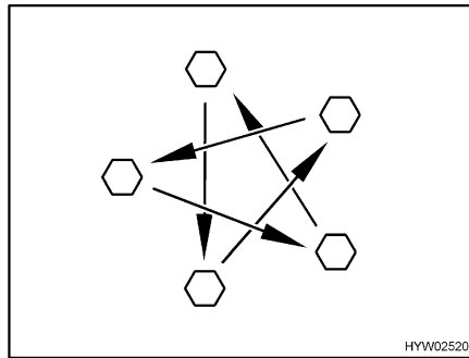
Afb. 186 Wielmoeren of wielschroeven kruisgewijs aandraaien
