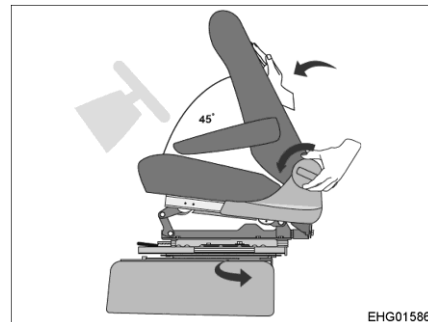
Afb. 24 De rugleuning naar voren kantelen
