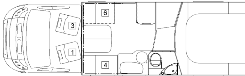
Afb. 19 Zitplaatsen
