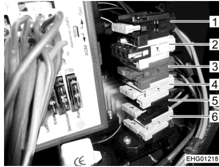
Afb. 126 Zekeringen naast het elektro-blok (Ford)
