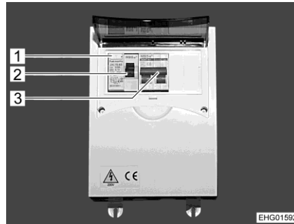
Fig. 134 Scatola dei fusibili a 230 V con interruttore di sicurezza e RCD (interruttore principale)
