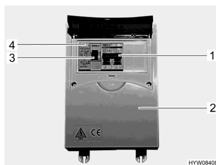
Fig. 116 Scatola dei fusibili a 230 V con interruttore di sicurezza e RCD (interruttore principale)
