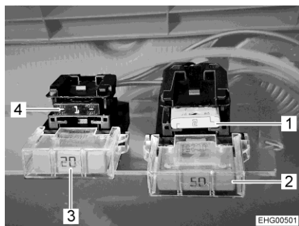
Fig. 123 Fusibili sulla batteria dell'abitacolo con booster di-ricarica (Stellantis)
