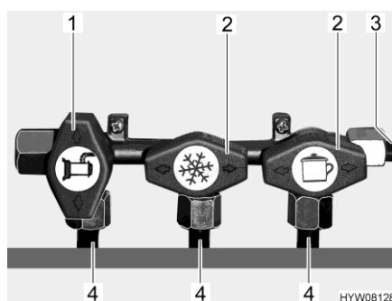
Fig. 111 Posizione dei rubinetti di arresto del gas (esempio)
