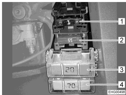
Fig. 121 Fusibili sulla batteria di avviamento con booster di ricarica
