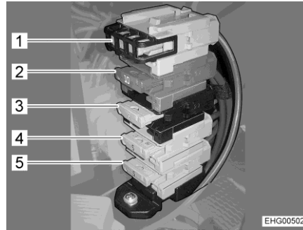
Fig. 127 Fusibili accanto alla centralina elettrica con predisposizione per pannello solare e impianto satellitare
