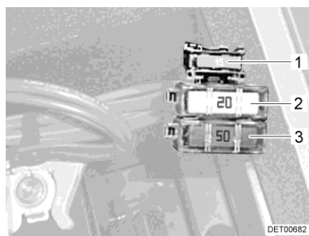
Fig. 120 Fusibili sulla batteria di avviamento senza booster di ricarica
