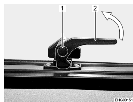
Fig. 49 Leva di serraggio, inferiore (posizione "Chiuso")
