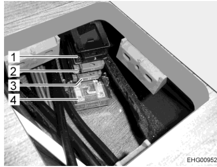
Fig. 124 Fusibili sulla batteria di batteria dell'abitacolo con booster di ricarica (Ford)
