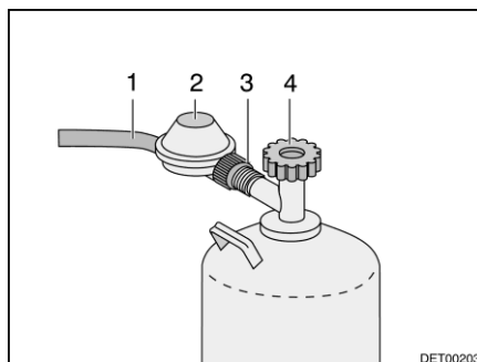
Fig. 109 Raccordo bombola del gas
