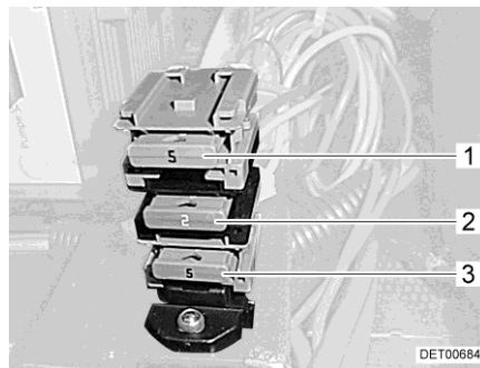
Fig. 125 Fusibili accanto alla centralina elettrica (Stellantis)
