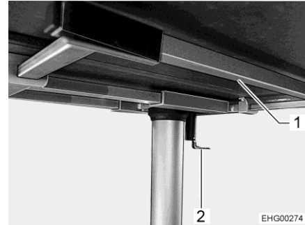
Fig. 74 Lato inferiore del tavolo
