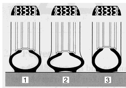
Fig. 187 Base di appoggio degli pneumatici
